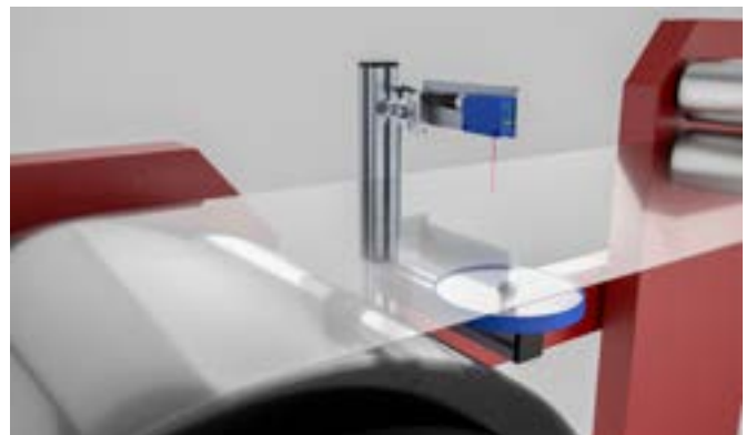
Detekce transparentních fólií je problematická. V případě ultrazvukových závor a nedostatečně napnutého snímaného materiálu se může stát, že ultrazvukový impulz vysílače skrze molekuly vzduchu rozkmitá i snímanou fólii. Průběh signálu mezi vysílačem a přijímačem se proto nepřerušuje. Senzor OR270478 tento problém zcela eliminuje.
