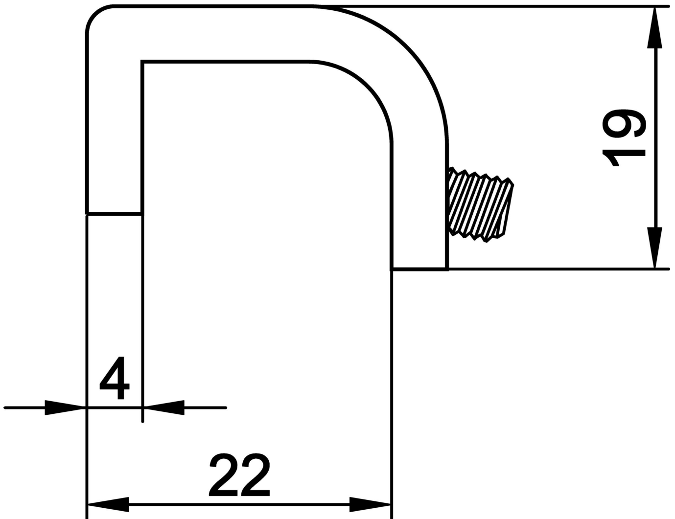
Rysunek wymiarowy
