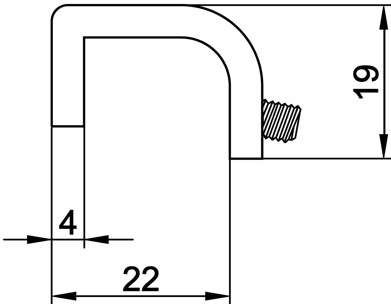
尺寸图
