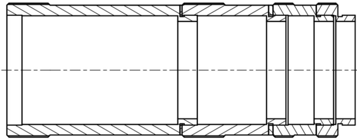
A-A ( 2 : 1 )
