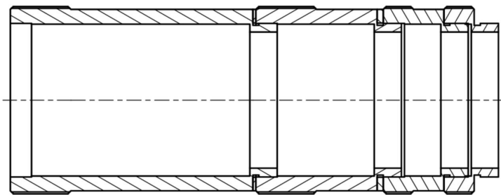
A-A ( 2 : 1 )
