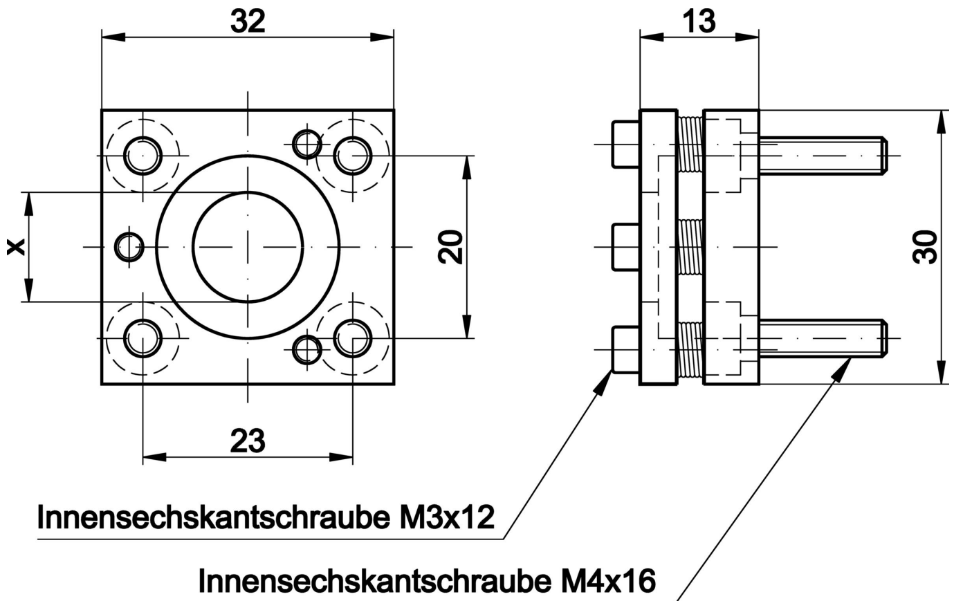
尺寸图
