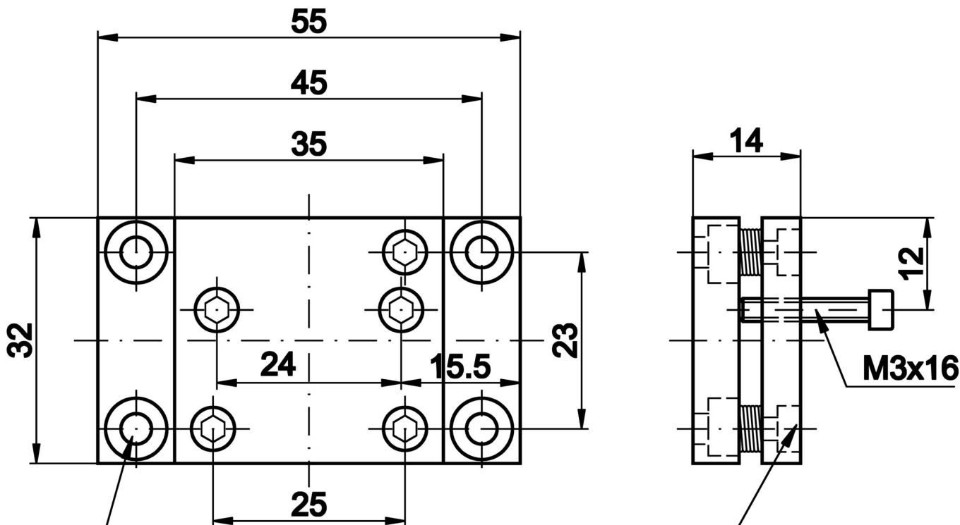
Innensechskant- schraube M4x10
