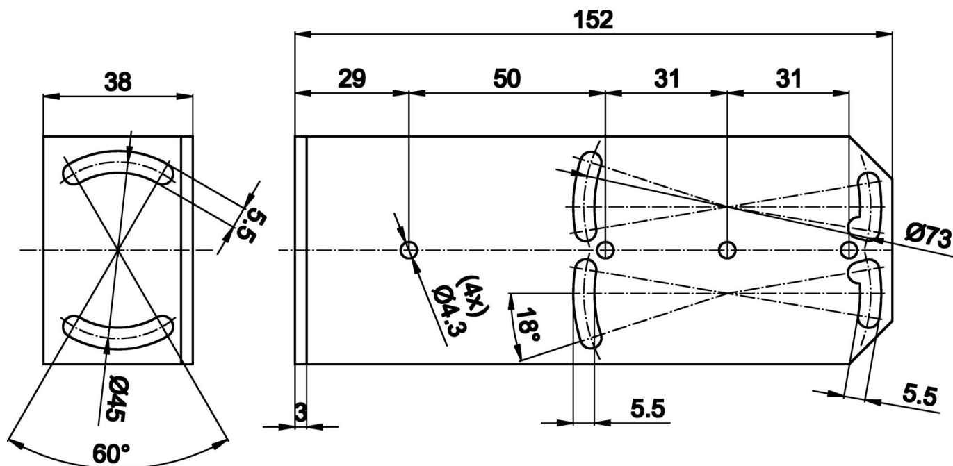
Rysunek wymiarowy
