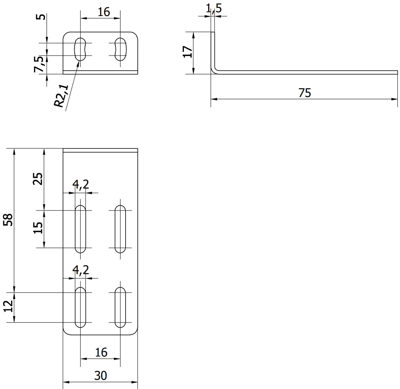
Rysunek wymiarowy
