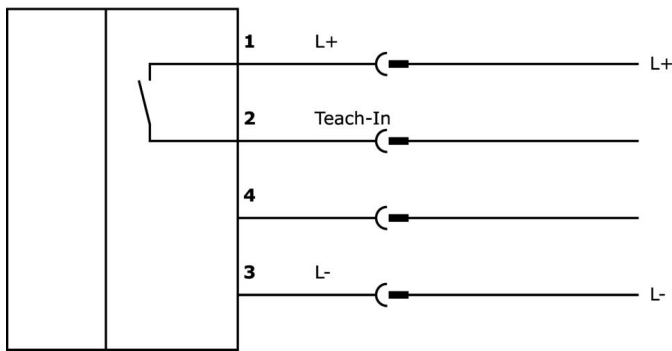
Adattatore didattico
