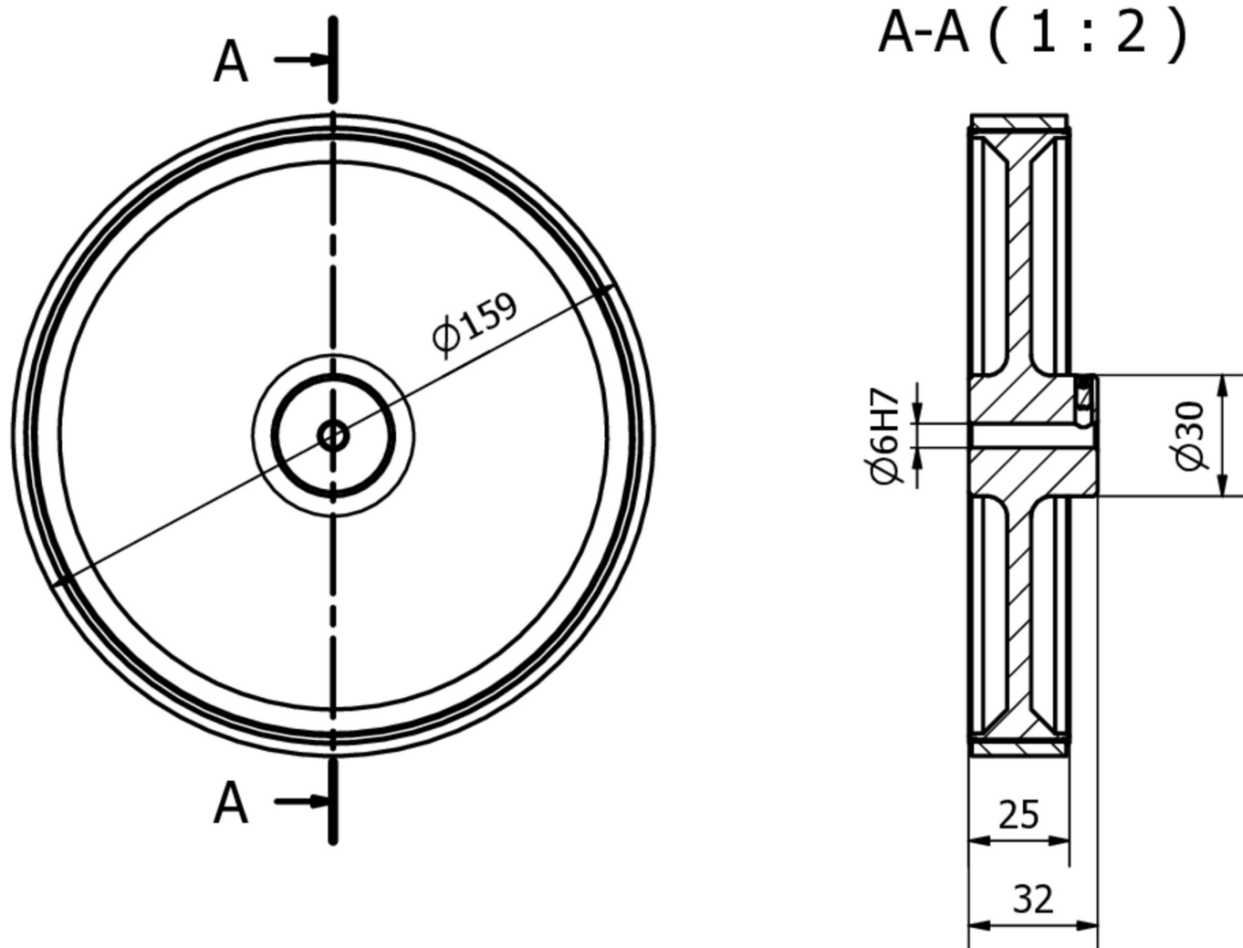
Rysunek wymiarowy
