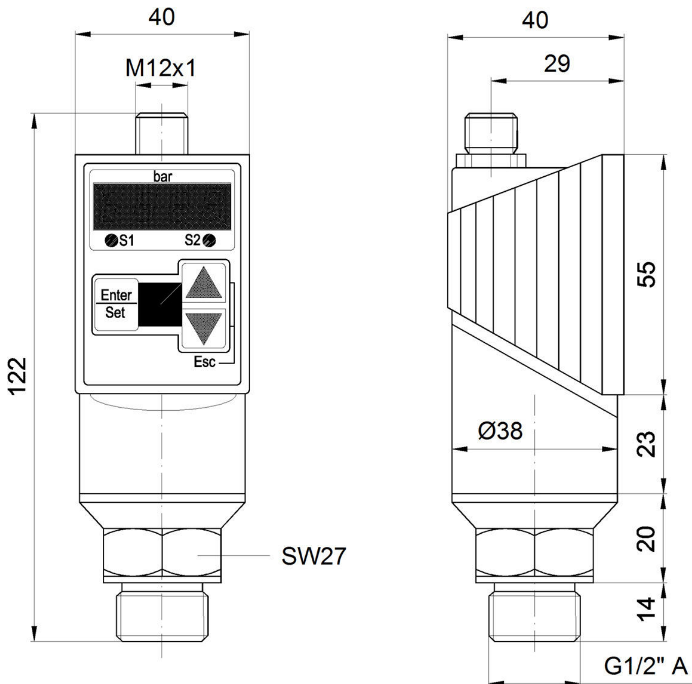
Rysunek wymiarowy
