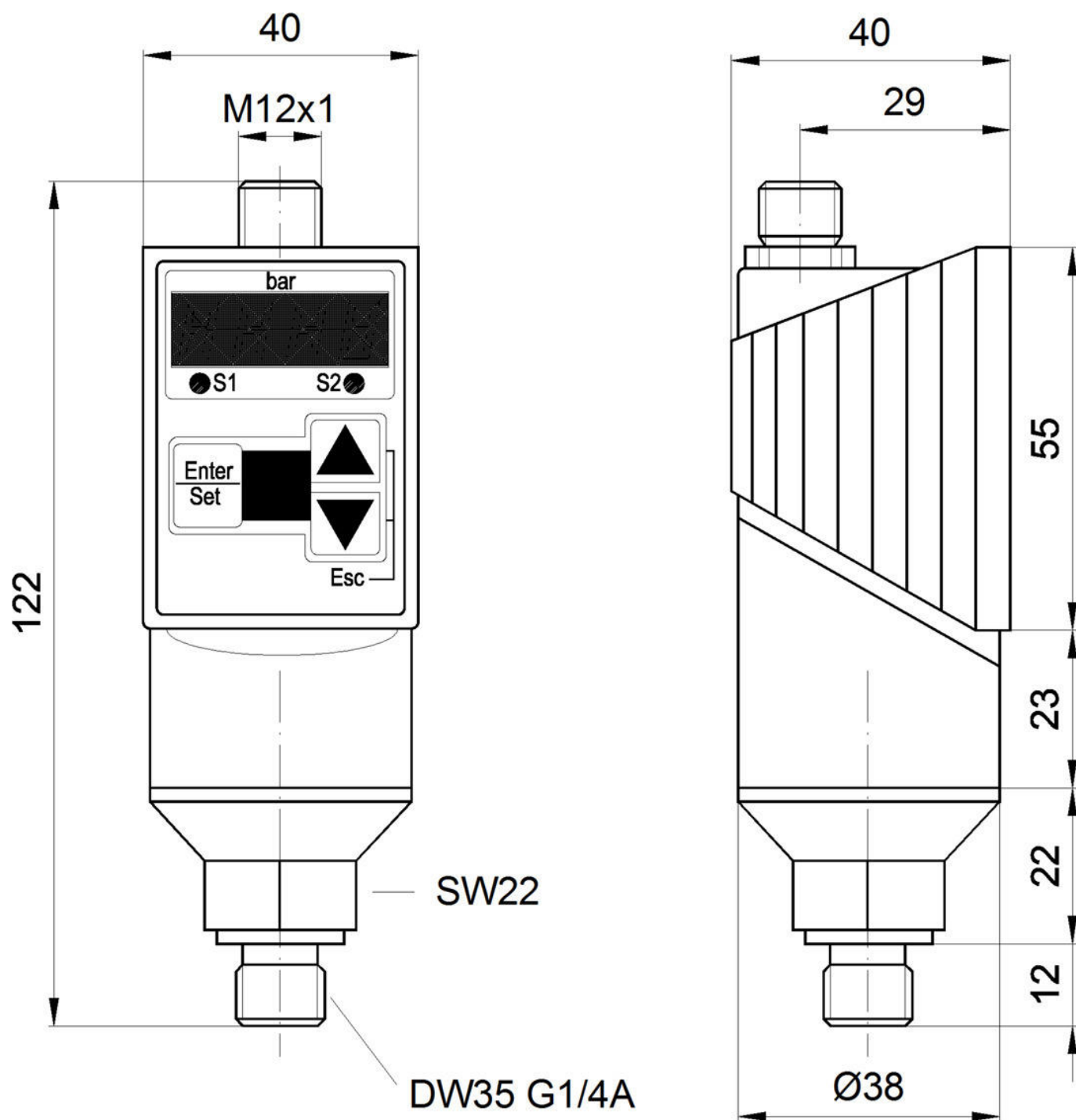
尺寸图
