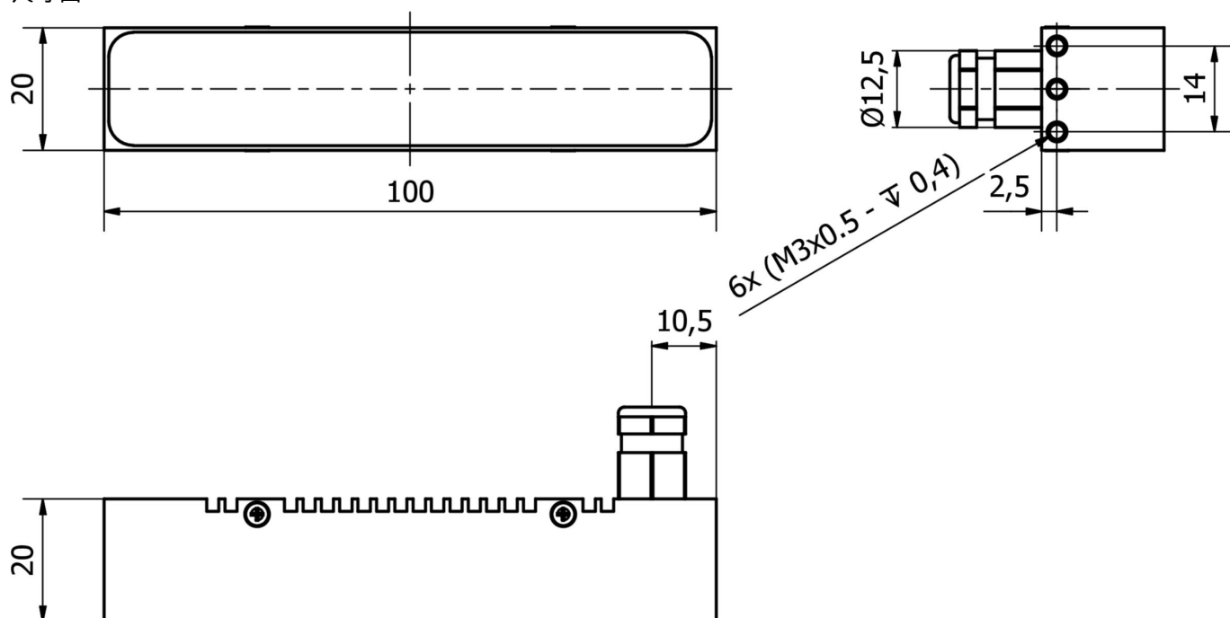
尺寸图
