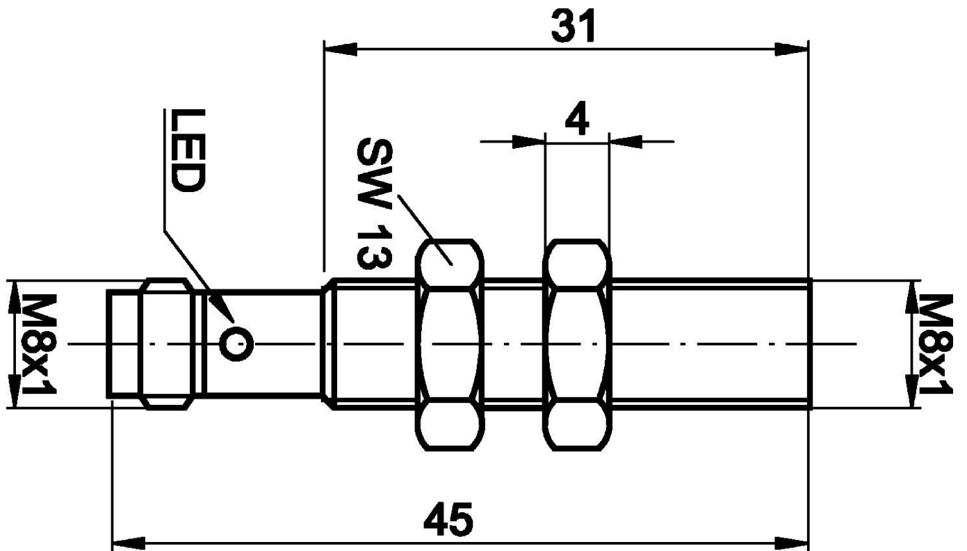
Rysunek wymiarowy
