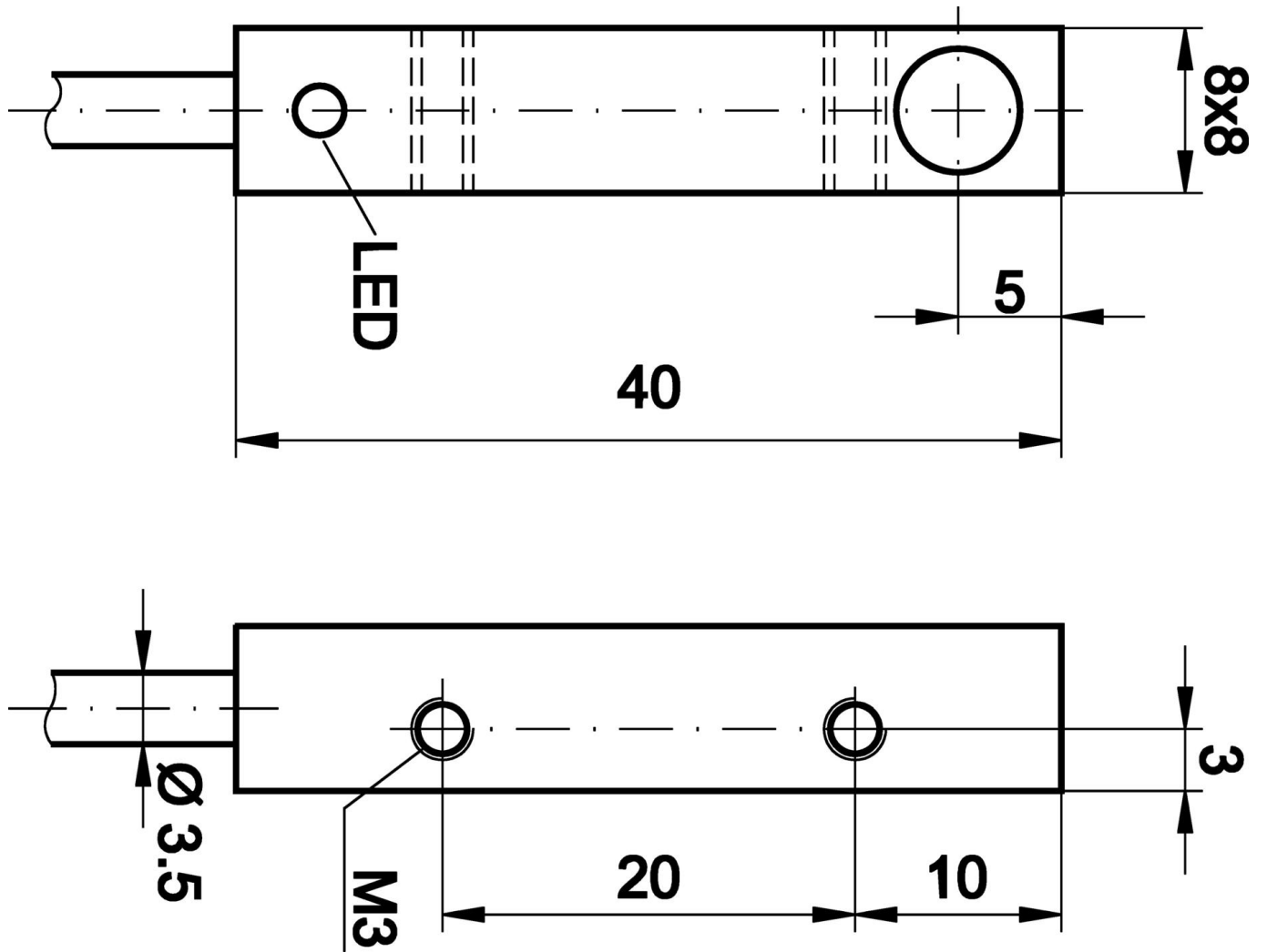
Rysunek wymiarowy
