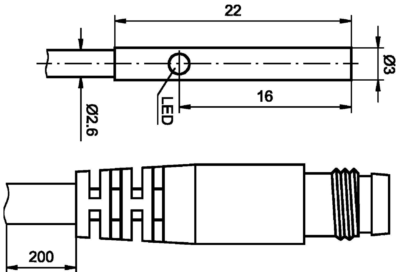
Rysunek wymiarowy
