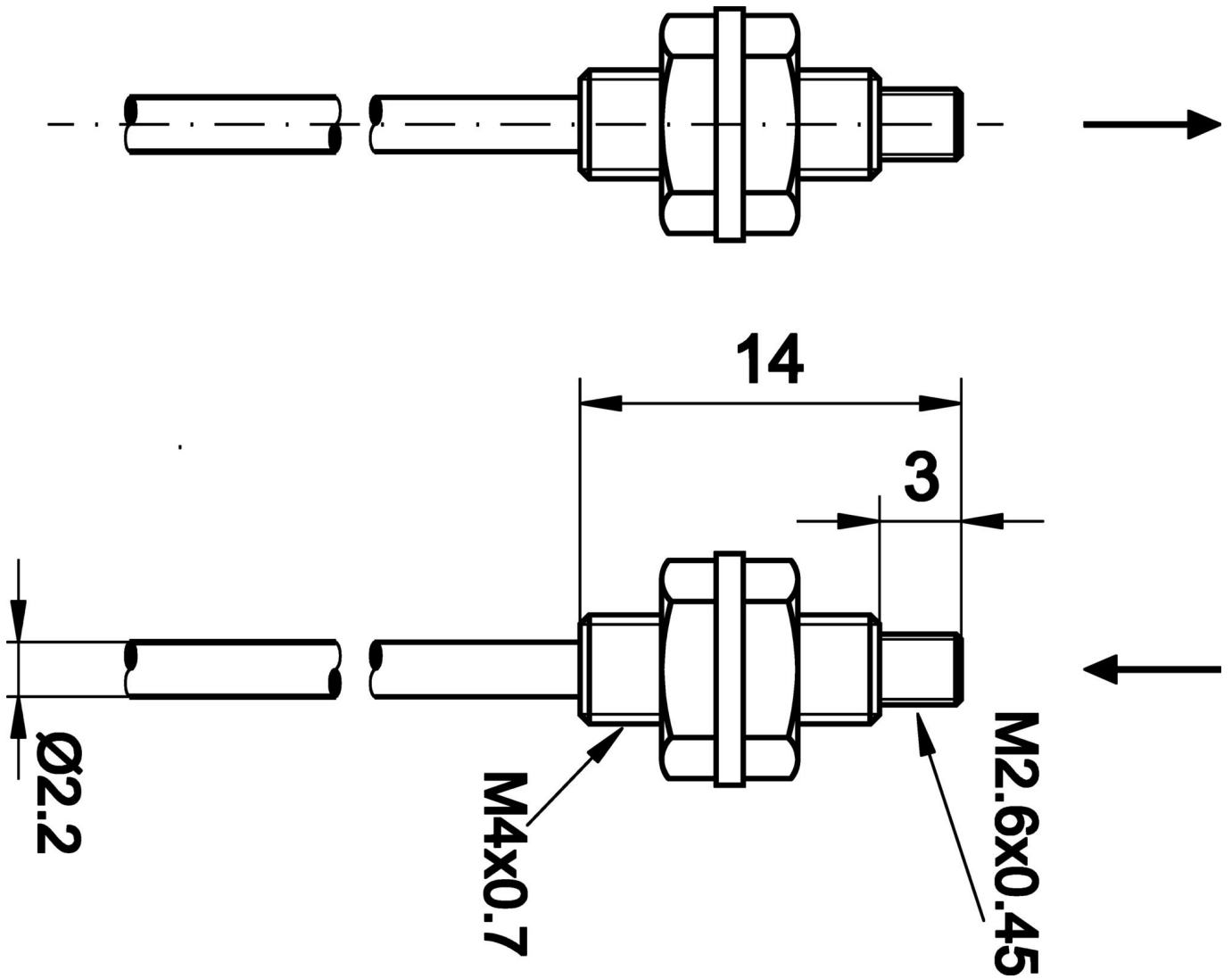
Rysunek wymiarowy
