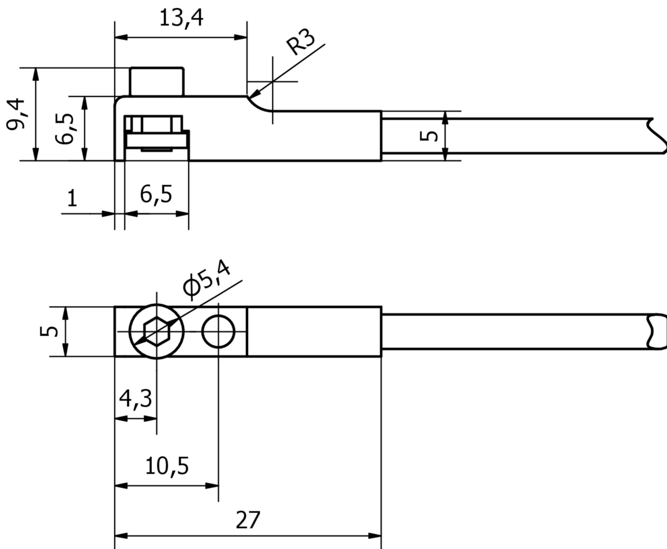
Rysunek wymiarowy
