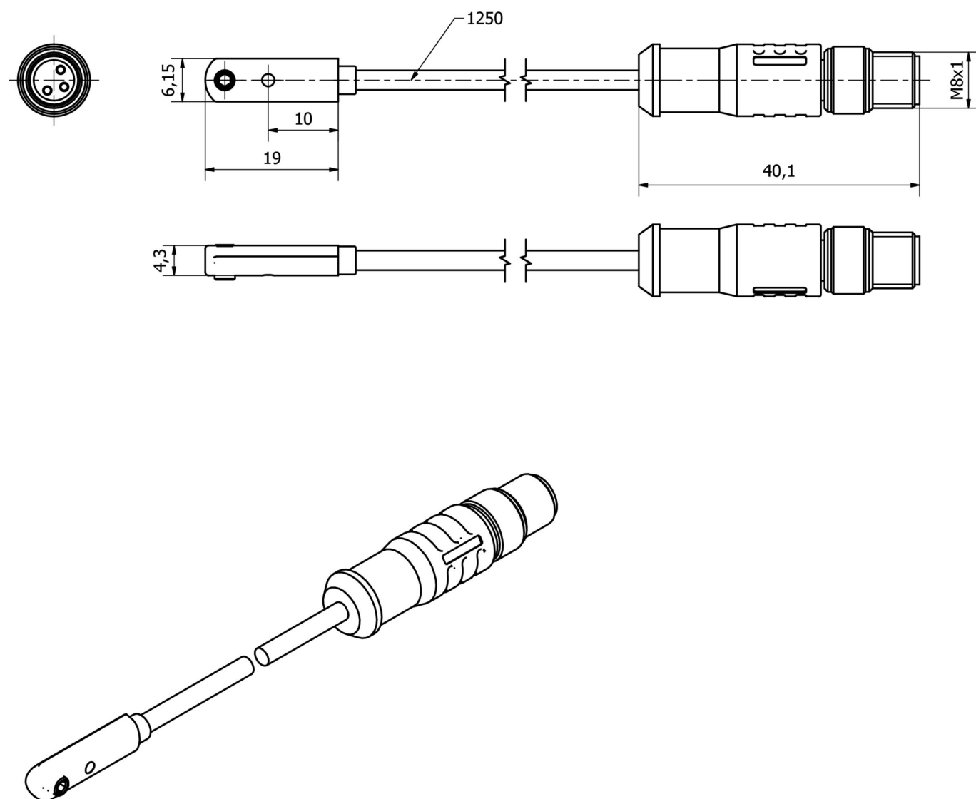
尺寸图
