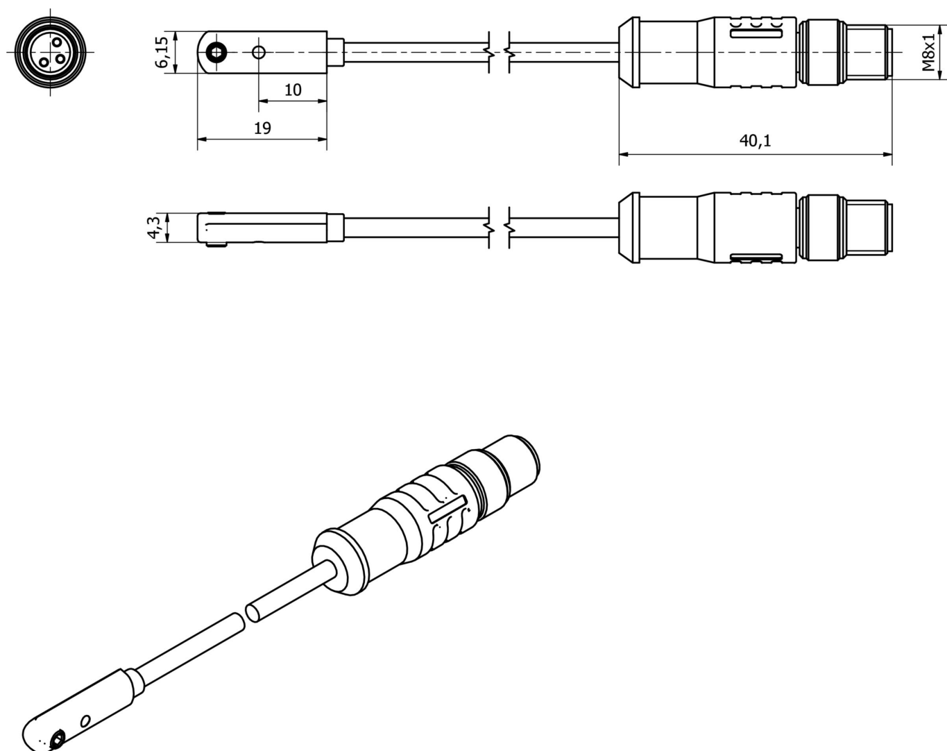
尺寸图
