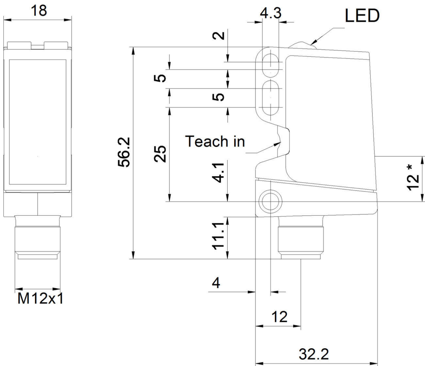
Rysunek wymiarowy
