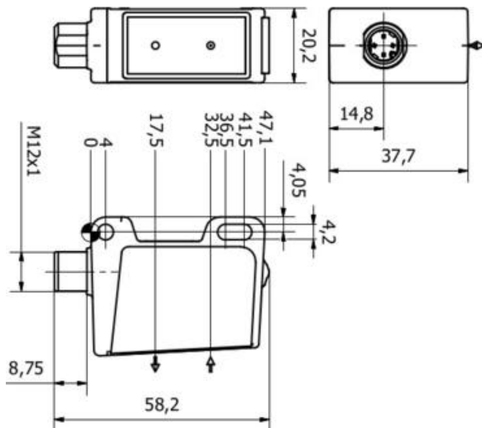
Rysunek wymiarowy
