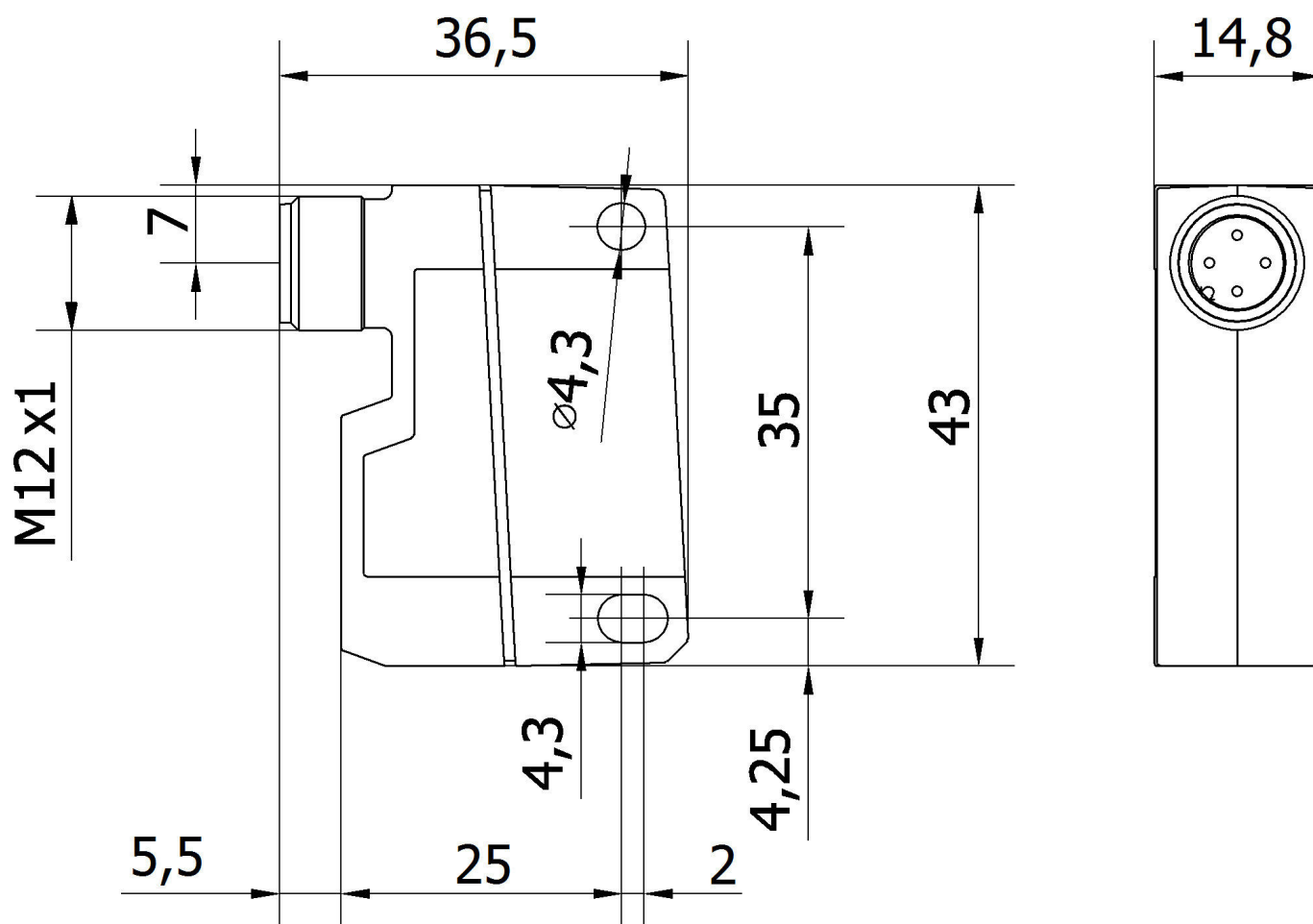
Rysunek wymiarowy
