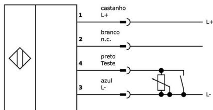
Entrada de teste: Transmissor desligado = 0V Potência de transmissão ajustável através de um potenciómetro de 10KΩ
