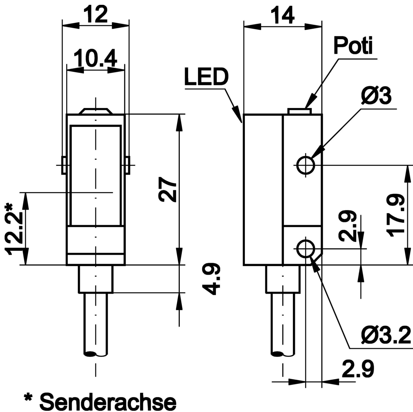
尺寸图
