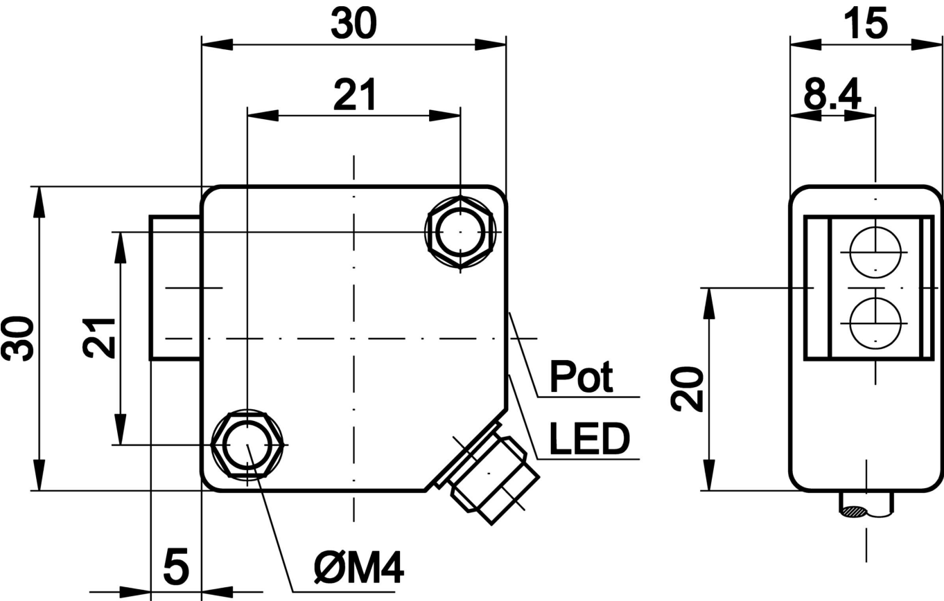
尺寸图
