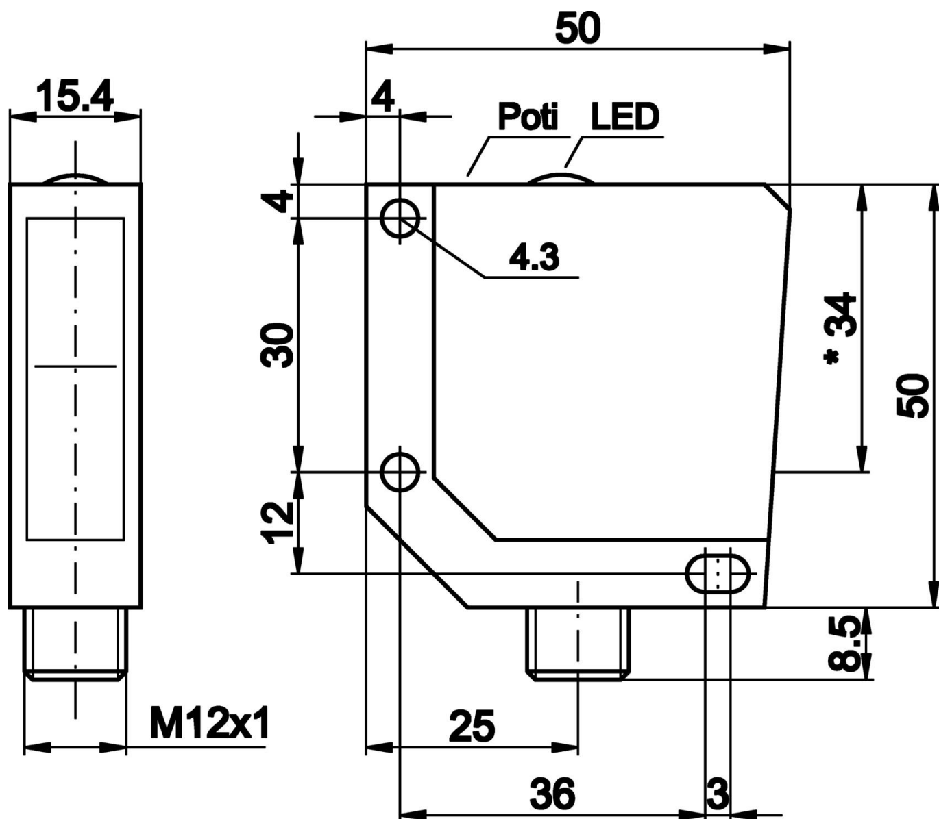
尺寸图
