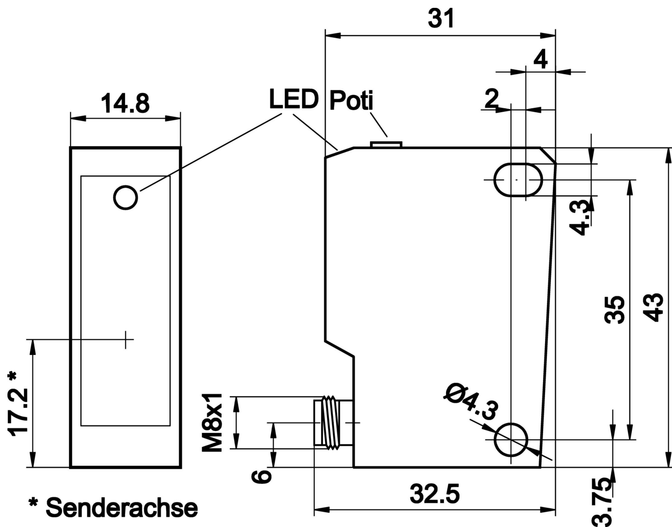
尺寸图
