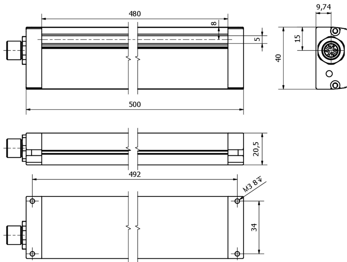
Rysunek wymiarowy
