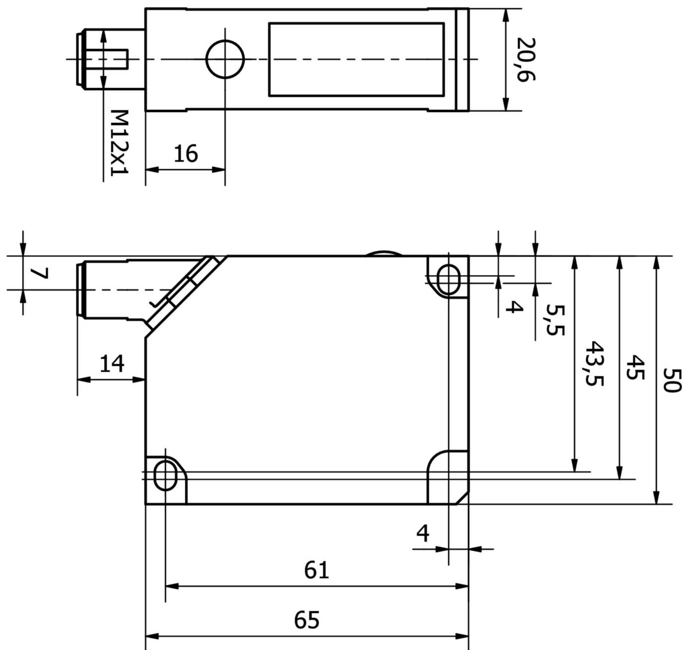
Rysunek wymiarowy
