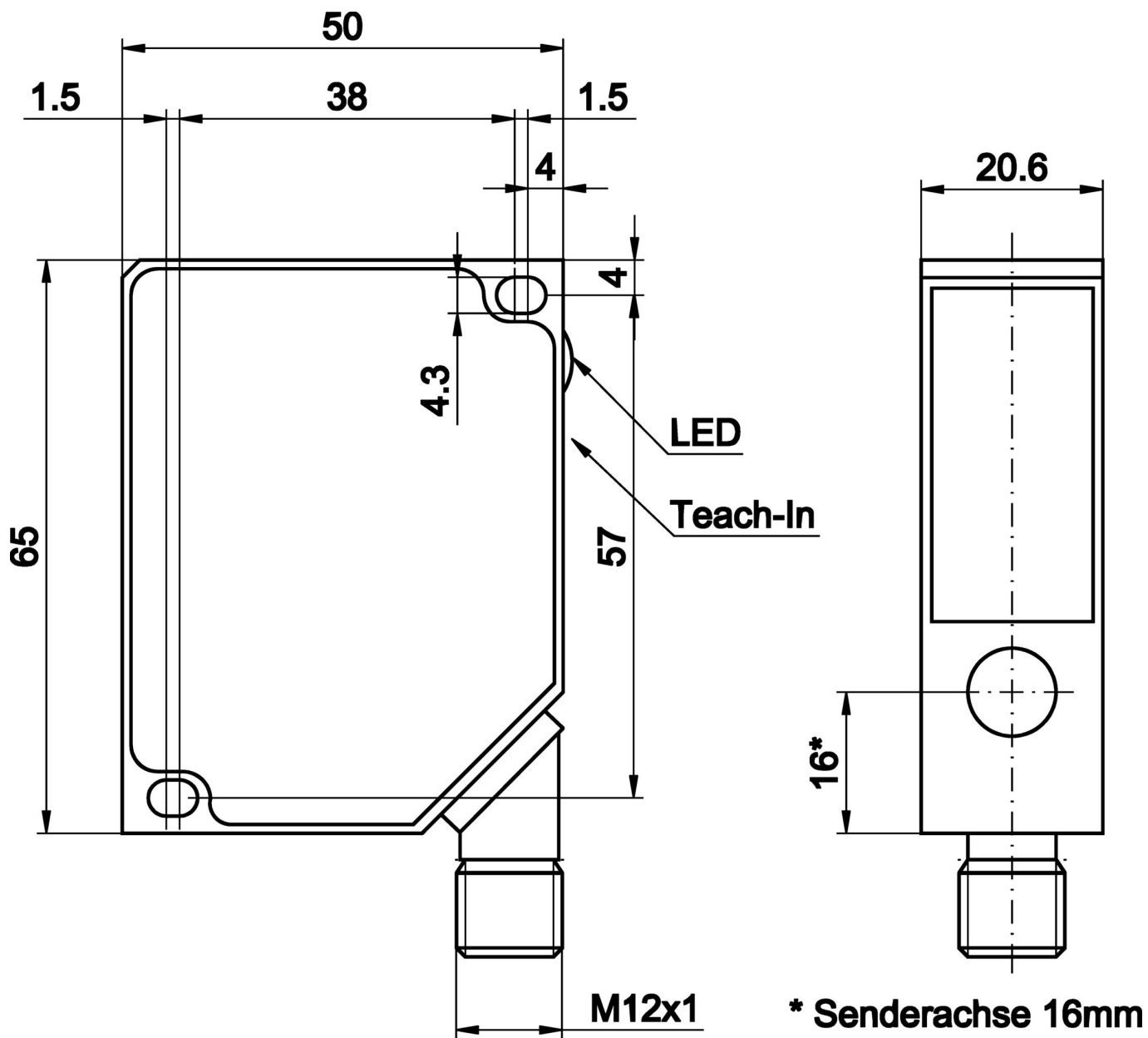
Rysunek wymiarowy
