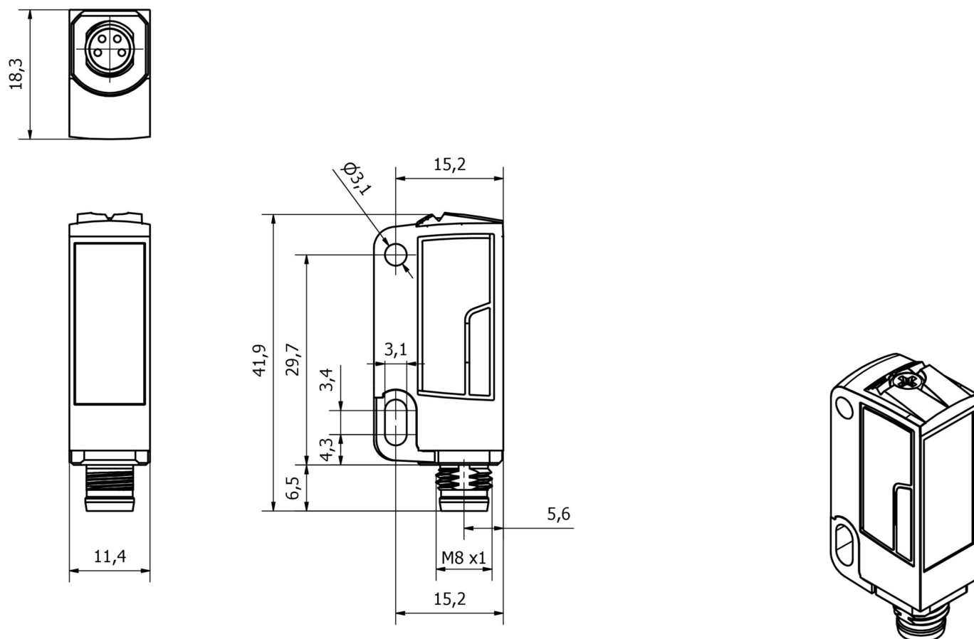
Rysunek wymiarowy
