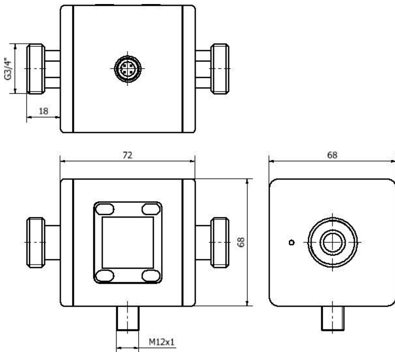
尺寸图
