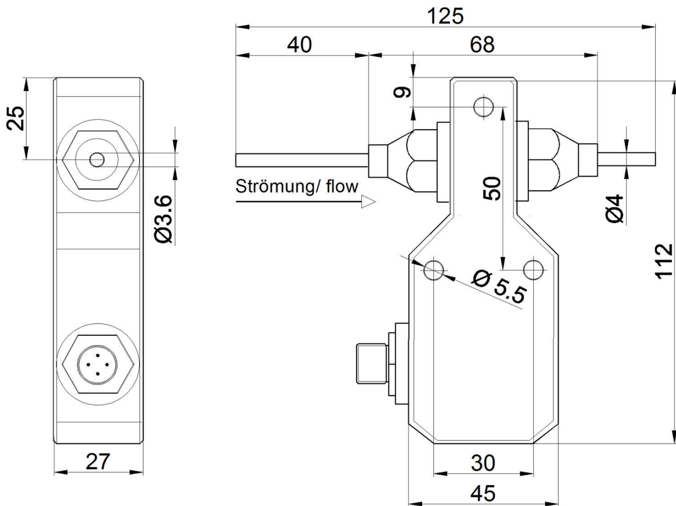
Rysunek wymiarowy
