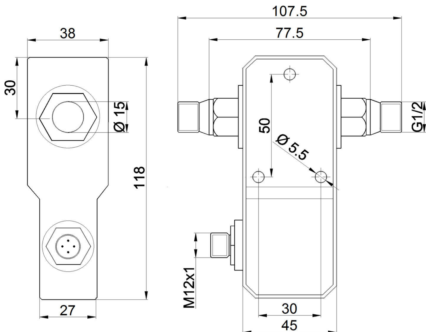
尺寸图
