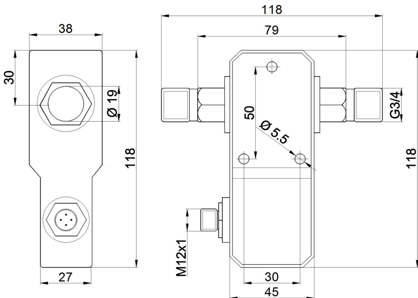
尺寸图
