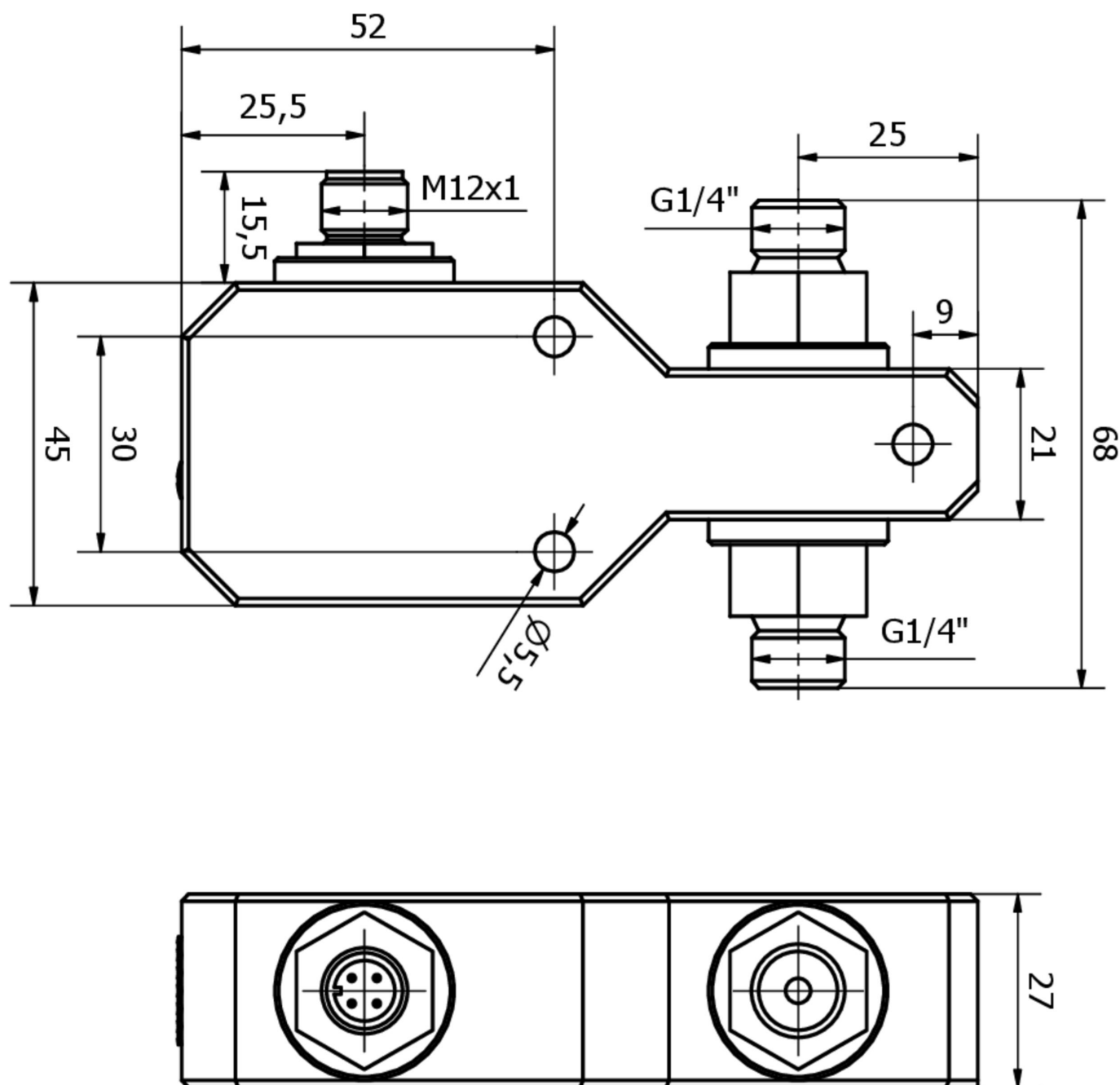
尺寸图
