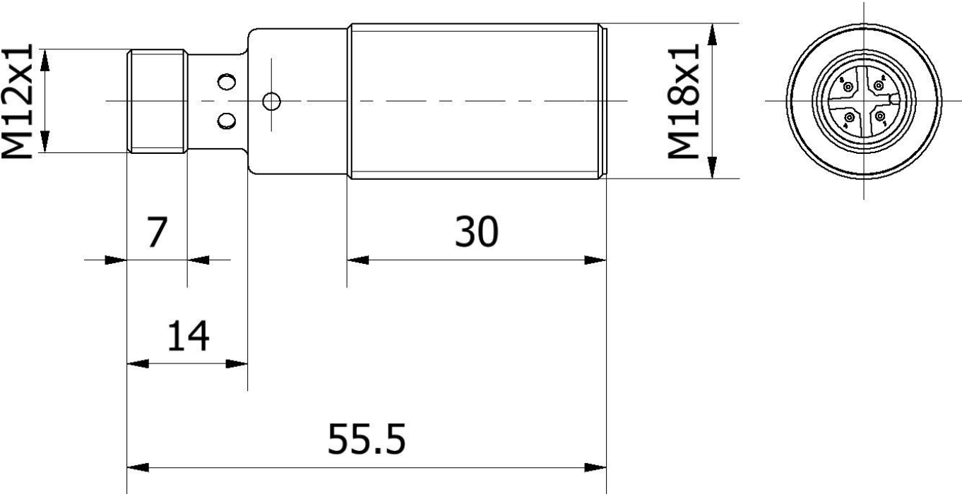
尺寸图
