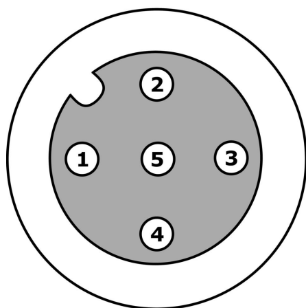
Prise femelle
