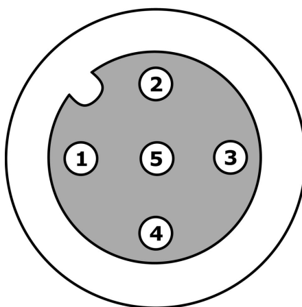
Prise femelle
