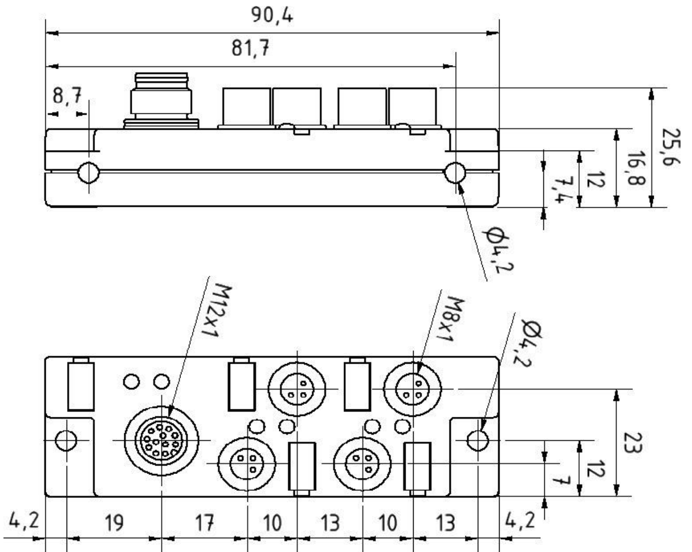
Rysunek wymiarowy
