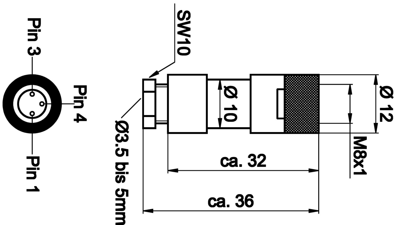
Rysunek wymiarowy
