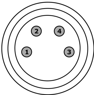
Zástrčka
