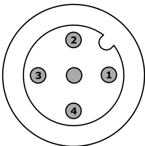
Zástrčka
