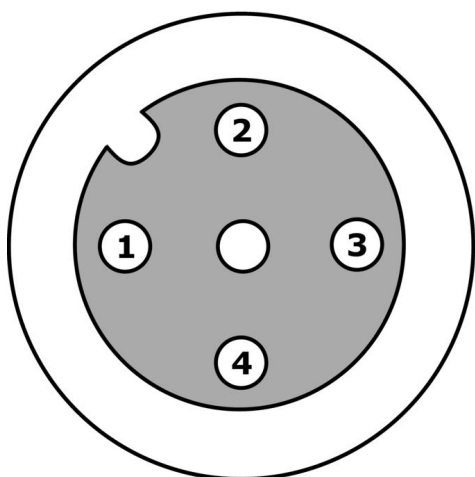
Zásuvka
