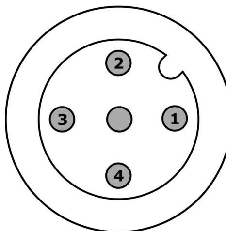
Zástrčka
