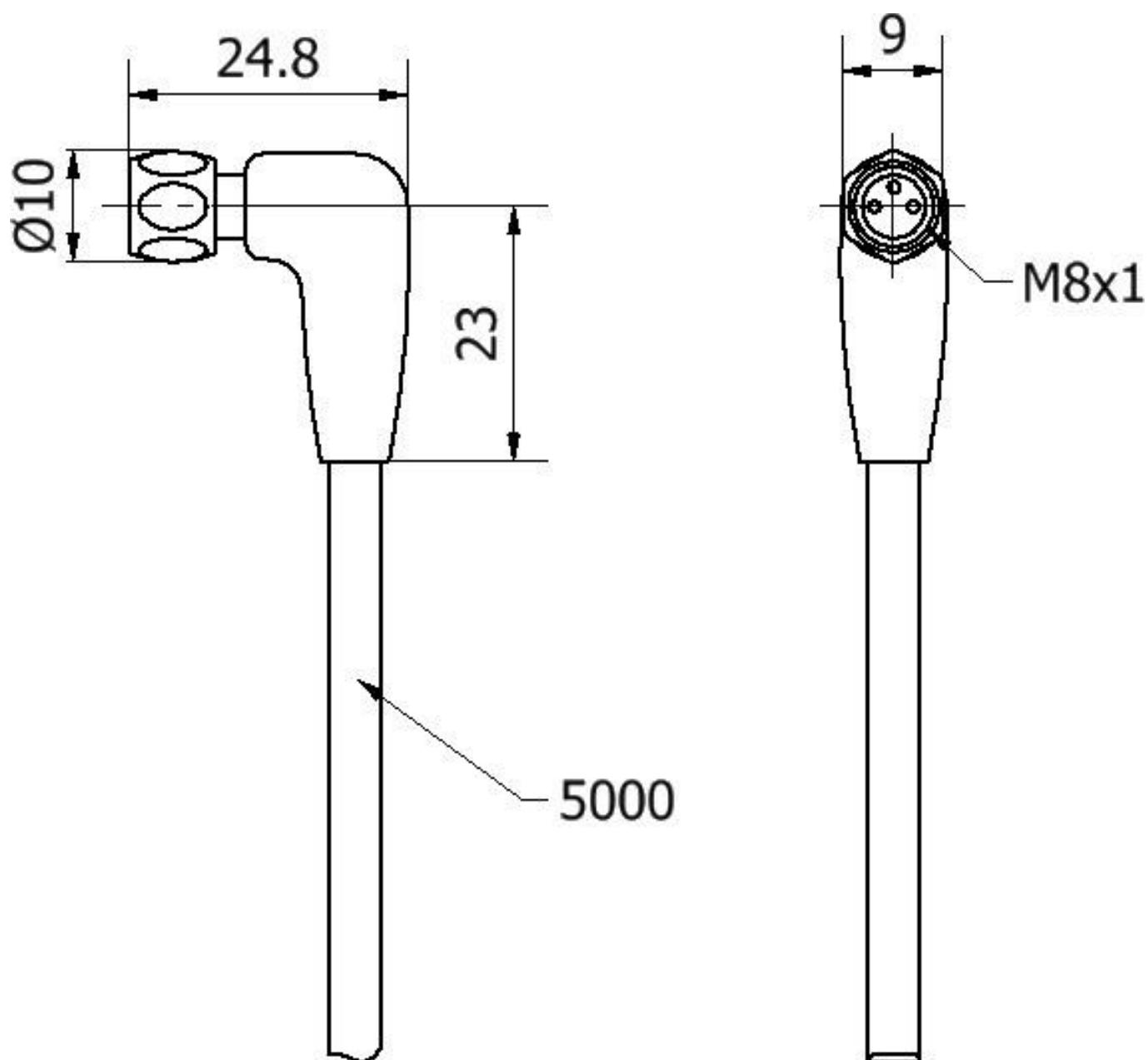
尺寸图
