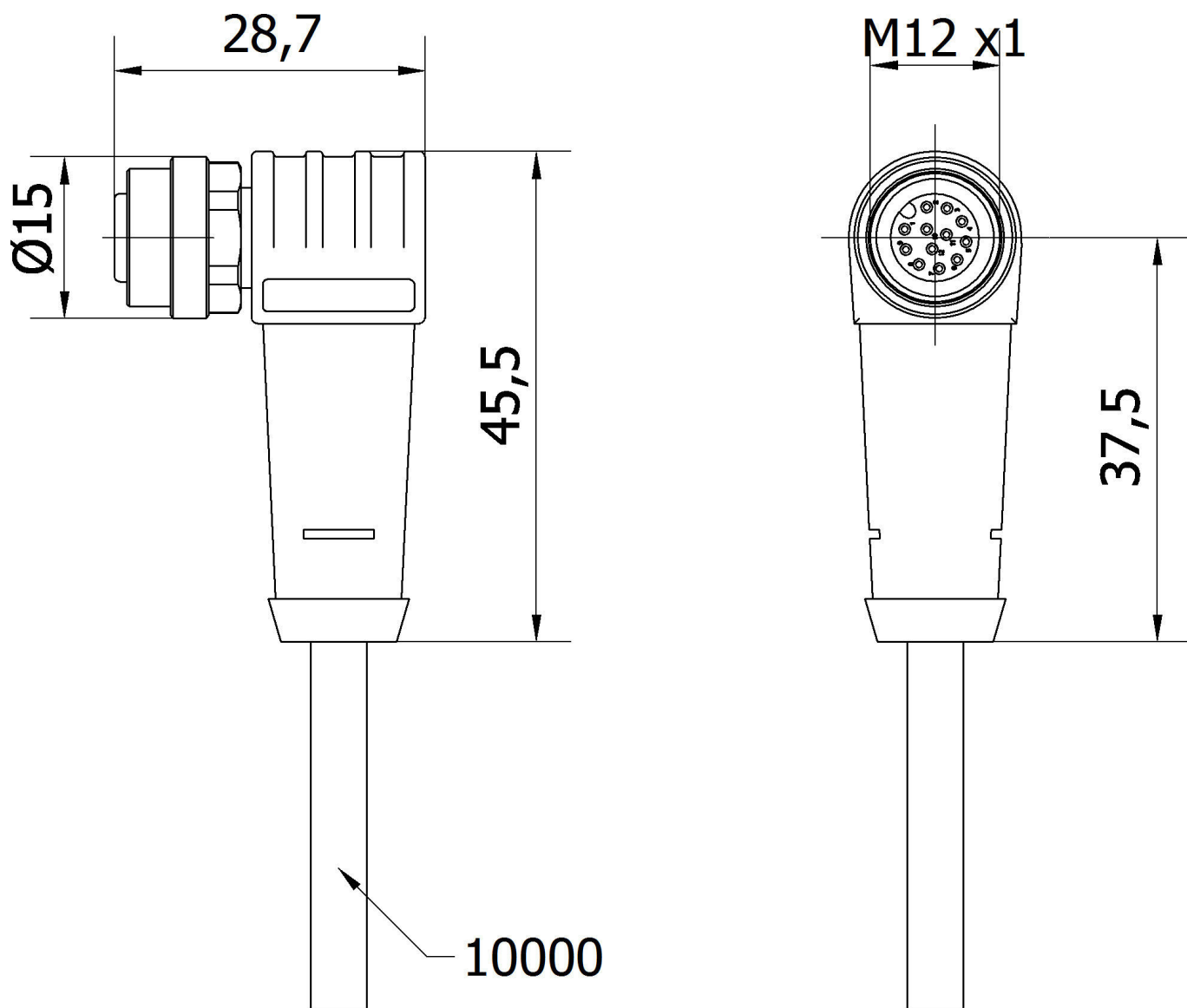
Rysunek wymiarowy
