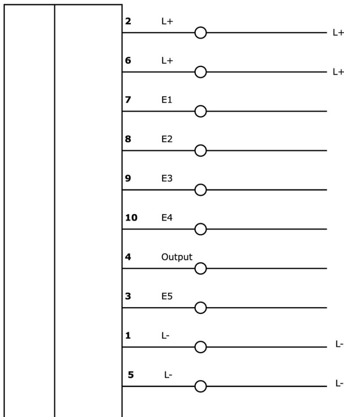
ODER-Modul
