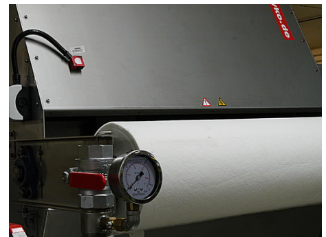
Einlaufseite des Filtervlieses: Ein optischer Taster von ipf electronic überwacht mit einem permanent anstehenden Signal das Vorhandensein des Filtervlieses. Ist das Filtervlies verbraucht, fällt das Signal vom Sensor ab und meldet somit der SPS der Anlage, dass neues Vlies eingelegt werden muss.
