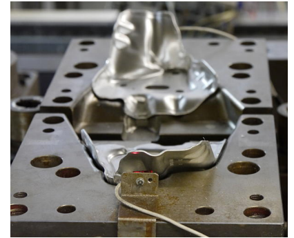
Vysoká provozní bezpečnost: V různých stanicích progresivního lisu jsou integrovány optické senzory, které zjišťují, zda jsou plošné spoje správně situovány pro následné zpracování.
