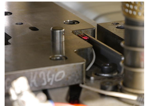
Díky jeho rozměrům je možné snímač pro kontrolu posuvu instalovat přímo do lisovacích strojů.
