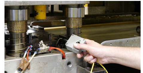
Snímač lze velmi snadno naučit zvenčí prostřednictvím Teachboxu, aniž by bylo nutné manipulovat se samotným snímačem.
